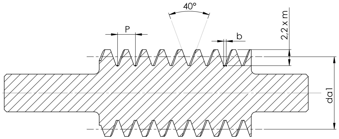
A-A (1 : 2)
